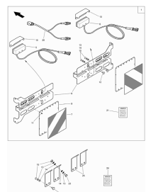
ETB-009187, Oświetlenie tylne
