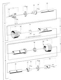
ETB-009183, Wałek przekąźnikowy, osłona wałka przekąźnikowego
