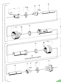
ETB-009184, Specjalny wałek przekąźnikowy ze sprzęgłem ciernym
