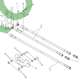
ETB-009185, Zespół dwudrogowy
