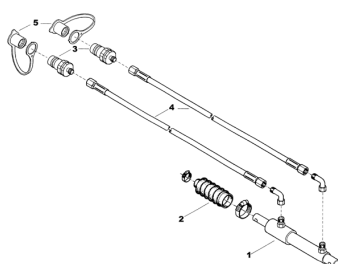
ETB-009175, Siłownik hydrauliczny
