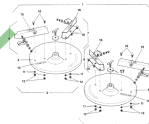
ETB-009170, Normalna tarcza rozsiewająca (czerwona)
