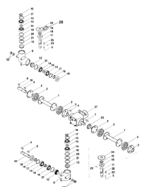
ETB-009171, Przekładnia kątowna
