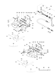
ETB-009174, Regulacja zasuw, siłownik hydrauliczny
