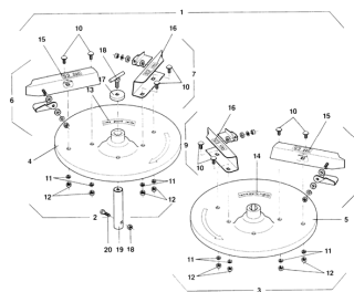
ETB-009180, Specjalna tarcza rozszewająca S4 kompl. (brązowa)
