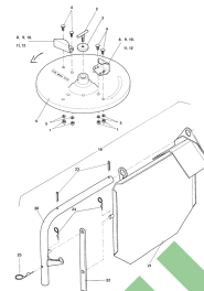
ETB-009181, Tarcza do rozszewu granicznego (zielona), ekran rozszewu granicznego
