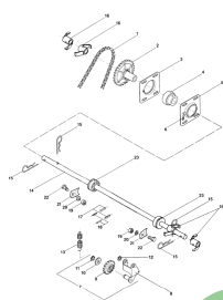
ETB-009172, Wałek mieszadła i jarzmo napinające do łańcucha
