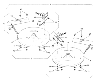
ETB-009178, Specjalna tarcza rozsiewająca S2 kompl. (szara)
