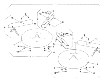
ETB-009177, Specjalna tarcza rozsiewająca S1 kompl. (pomarańczowa)
