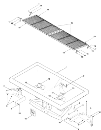
ETB-009167, Rama ze zbiornikiem kompl.
