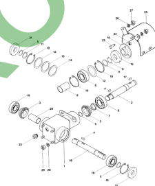
ETB-009173, Przekładnia wejściowa
