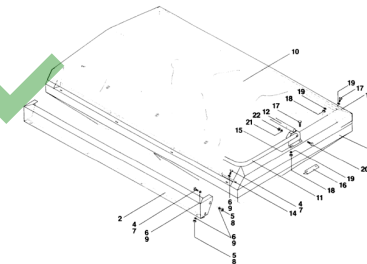
ETB-009182, Nadstawka nad zbiornik, plandeka
