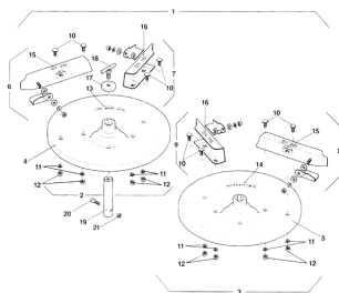
ETB-009179, Specjalna tarcza rozszewająca S3 kompl. (żółta)
